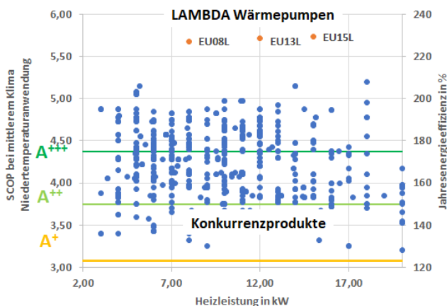
Účinnosť porovnávania trhu (SCOP) podľa EN 14825
